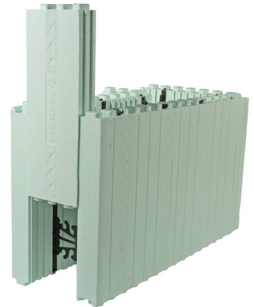
End Cap
